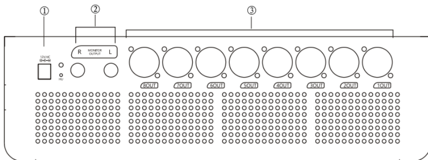
(Задняя панель микшера DM20M)
